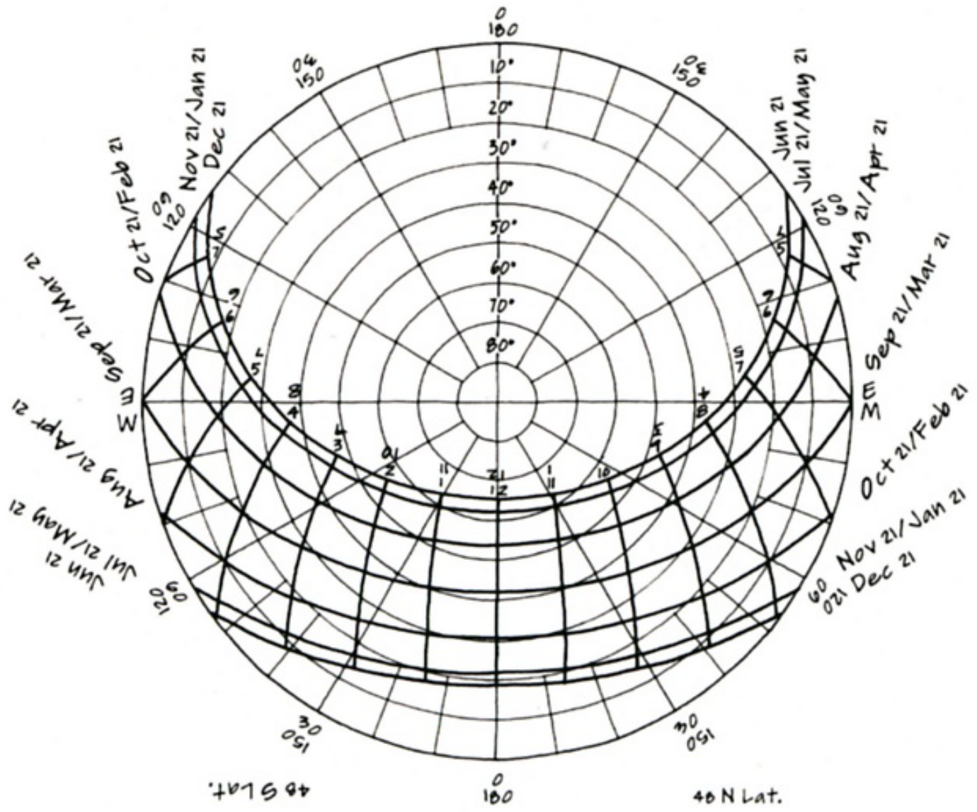
Sun Path Diagram, 40° Latitude
