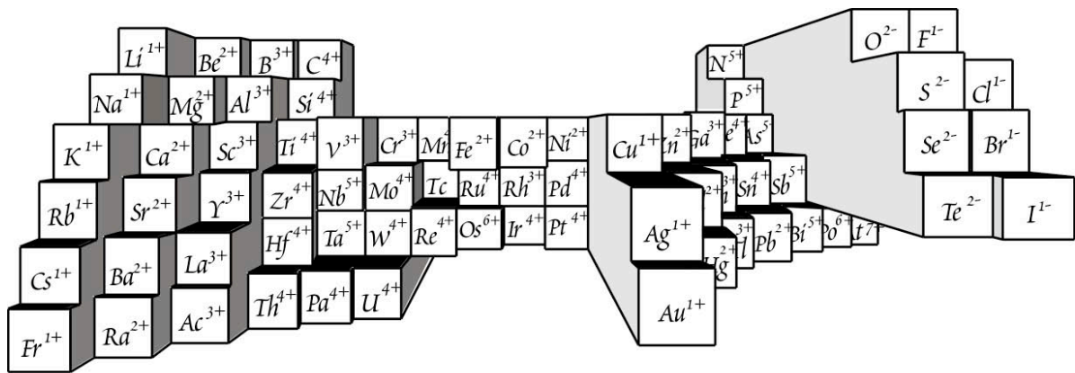
Ionic Radii
