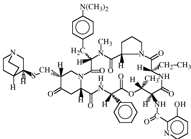
quinupristin
