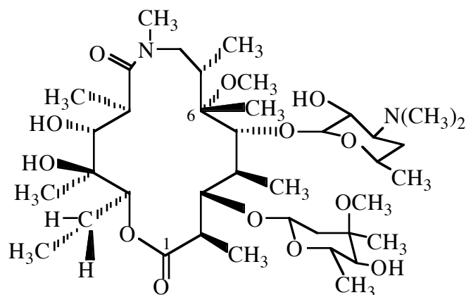
Azithromycin
