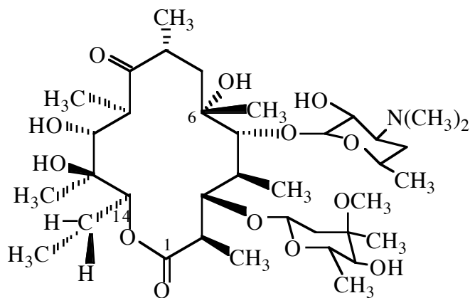
Erythromycin
