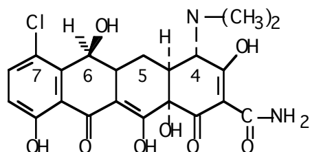
Demeclocycline
