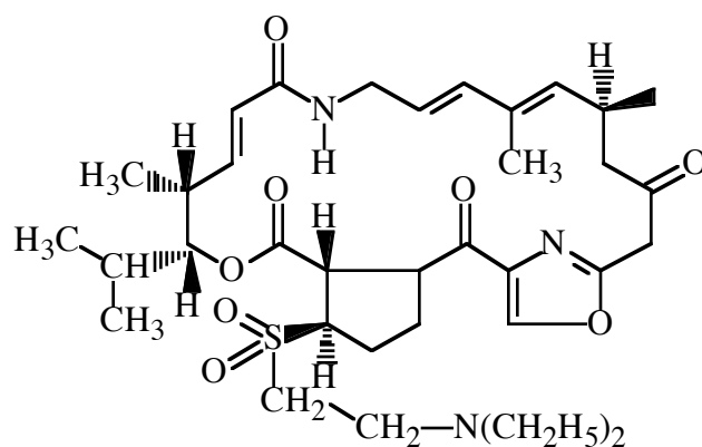
dalbapristin
