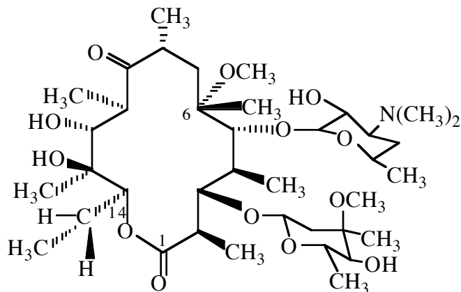
Clarithromycin
