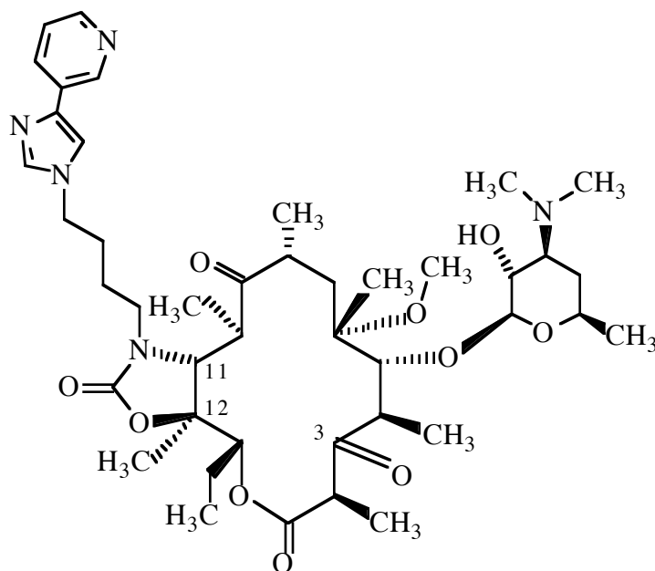
Telithromycin (Ketek®)
