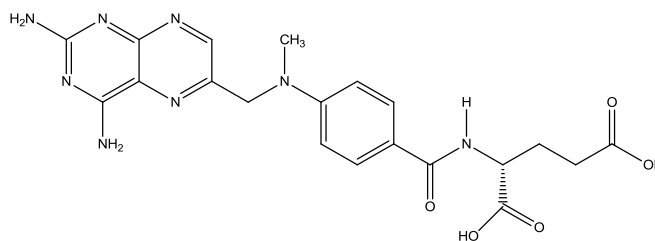
Methotrexate
